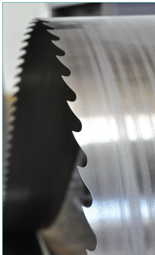
Danturare: Fiecare dinte este măsurat în mod automat pentru obținerea unei precizii maxime
